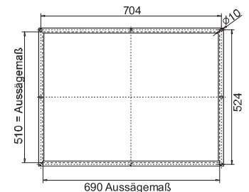
Einbaumaße Arbeitsplatte AK 6
